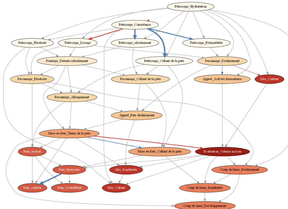
Figure 1 : Un exemple de modèle graphique d'apprentissage généré dans le projet EVAGRAIN
